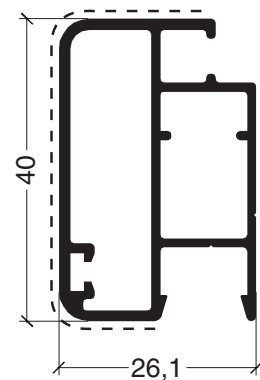
ADR 558 Mosq. reforzado 0,634 kg/m
