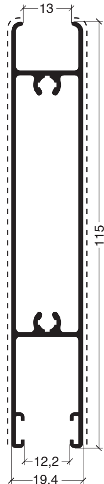
ADR 292 Zócalo alto /travesaño 1,081 kg/m
