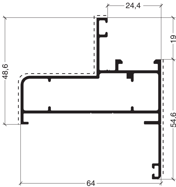
ADR 1513 Marco 64 mm con tapajuntas 0,952 kg/m
