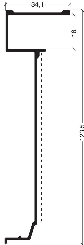
ADR 1381 Guía cortina barro 0,753 kg/m
