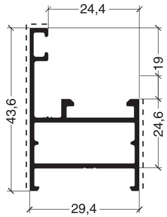
ADR 1161 Marco 29 mm 0,509 kg/m
