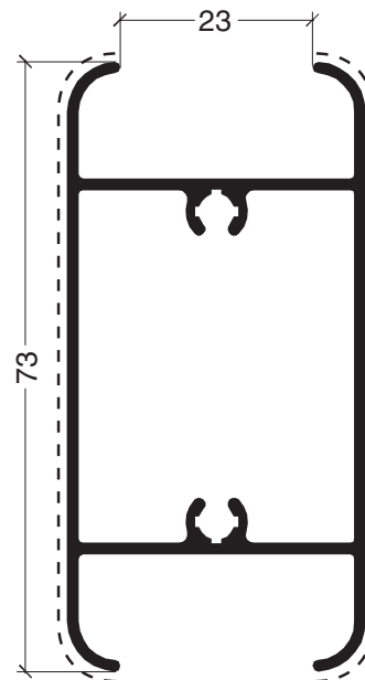
Escuadra AA256 Alineamiento AA 107
