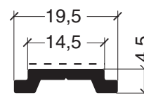
ADR 922 Pletina 0,139 kg/m
