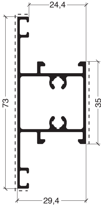
ADR 1168 Travesaño Paño Fijo 0,811 kg/m
