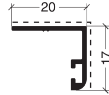
ADR 1164 Tapajuntas 0,145 kg/m
