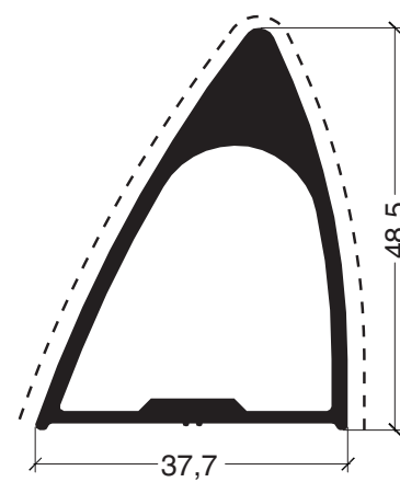
ADR 1515 Refuerzo de parante central 1,100kg/m
