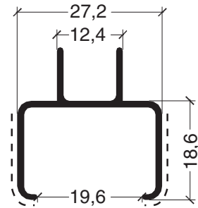
ADR 232 Adaptador para DVH 0,289 kg/m
