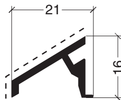
ADR 255 Vierendeel 0,201 kg/m
